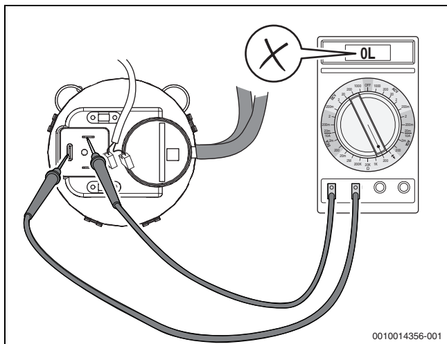
Рис. 70 Проверка проводимости дифференциального реле давления (реле неисправно )
