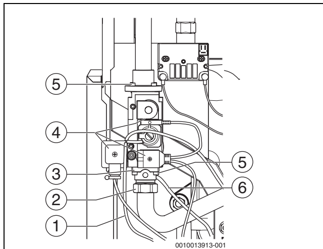
Рис. 59 Отсоединение подключений газовой арматуры (75 ... 100 кВт)
