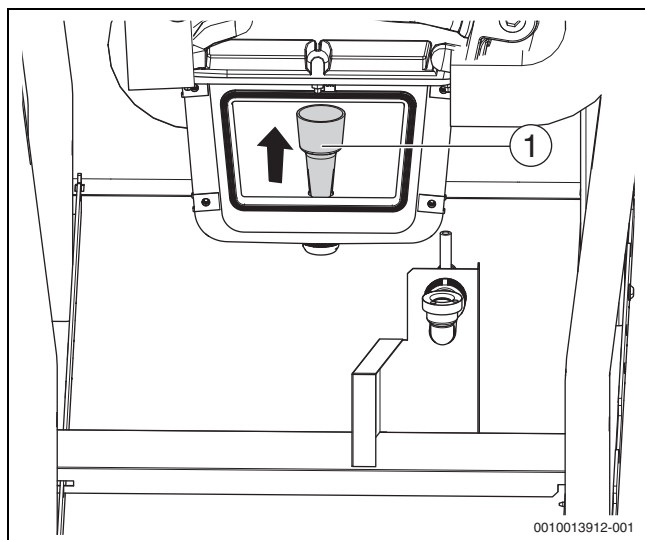
Рис. 50 Демонтированный грязеуловитель
