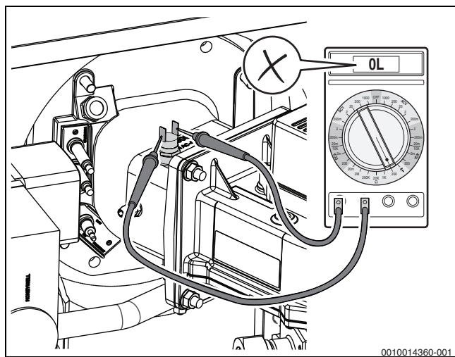
Рис. 66 Измерение электрического сопротивления на контактах реле контроля температуры (реле неисправно)
