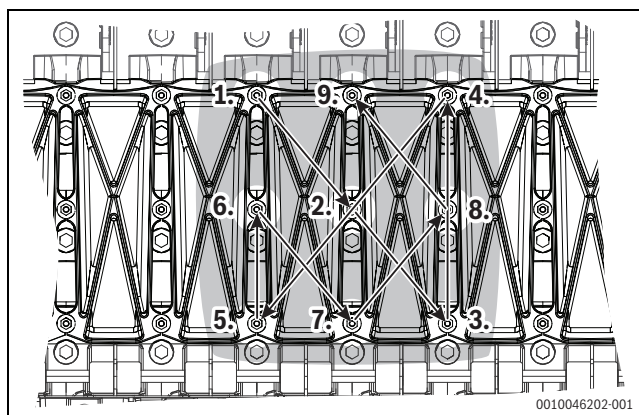
Рис. 55 Схема затяжки крышек люка для чистки
