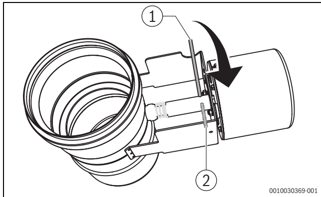
Рис. 29 Установочный штифт на запорном клапане
