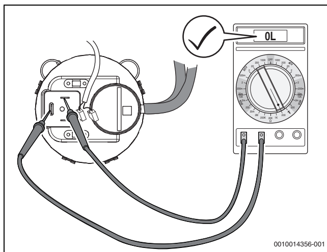
Рис. 71 Проверка проводимости дифференциального реле давления (реле в порядке)
