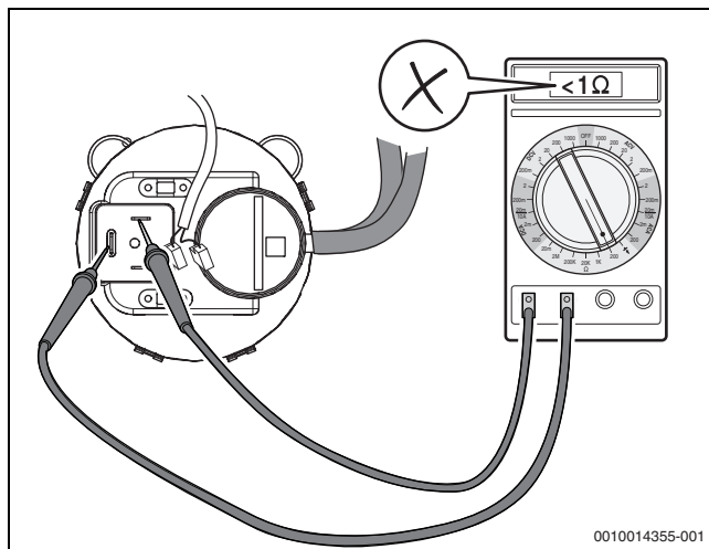
Рис. 72 Измерение электрического сопротивления на контактах дифференциального реле давления (реле неисправно )
