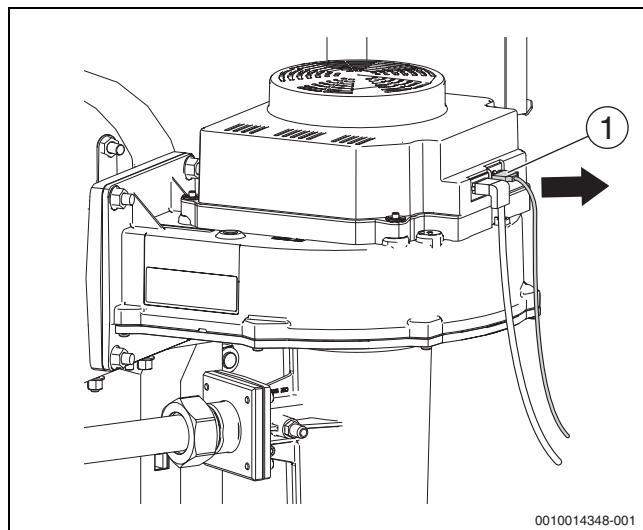
Рис. 67 Штекер сигнала PWM на вентиляторе (котлы 200-300 кВт)
