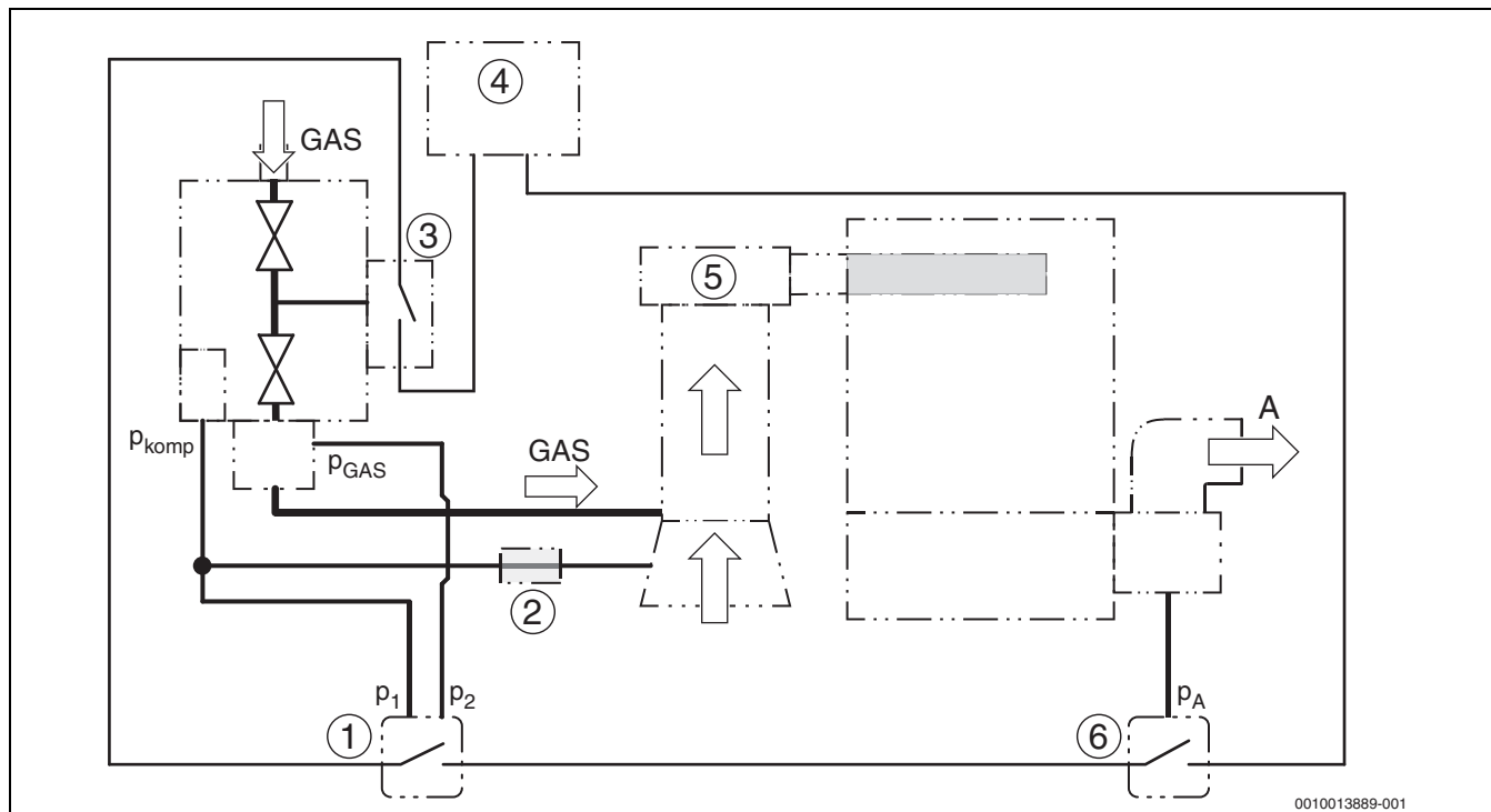
Рис. 75 Схема контроля приточного воздуха/отвода дымовых газов и утечек газа (по EN 15502)
