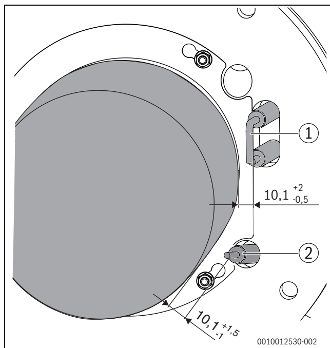
Рис. 57 Положение электродов (размеры в мм)
