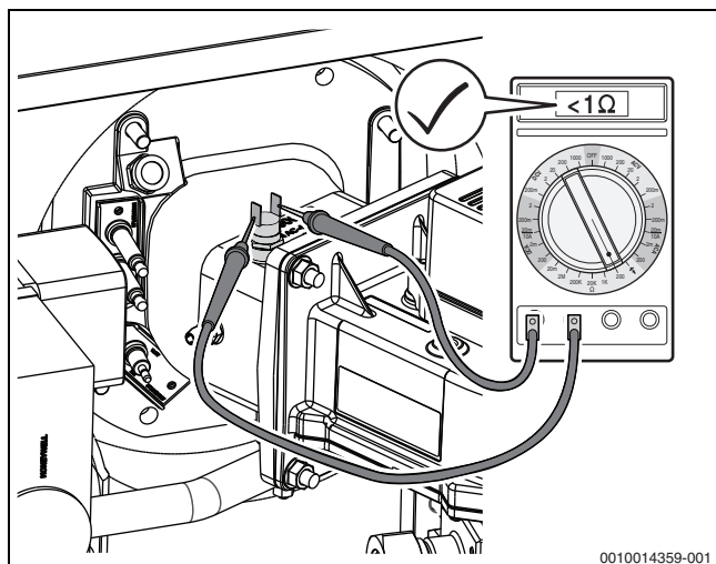
Рис. 65 Измерение электрического сопротивления на контактах реле контроля температуры (реле в порядке)
