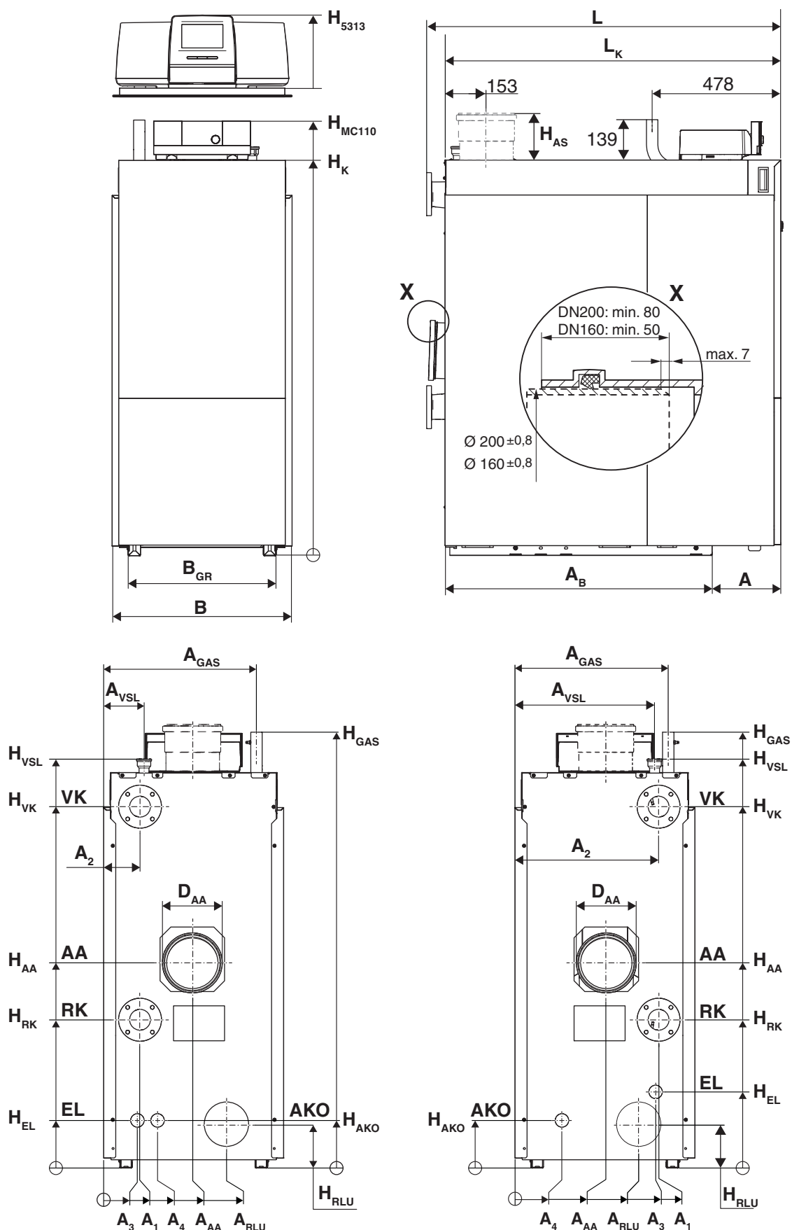
Рис. 4 Размеры и подключения для Logano plus KB372, 150...300 кВт (правое и левое исполнение; размеры в мм)
