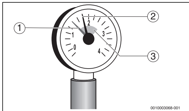
Рис. 38 Манометр для закрытых установок
