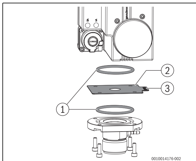
Рис. 26 Замена диафрагмы
