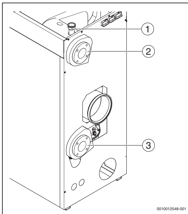
Рис. 15 Гидравлические подключения на котле (показан котёл с фланцевыми соединениями, правое исполнение)
