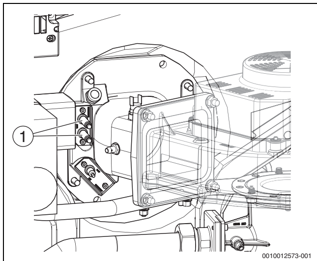
Рис. 39 Запальные электроды
