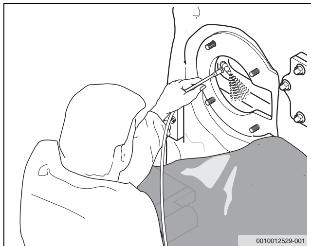
Рис. 56 Мокрая чистка теплообменника
