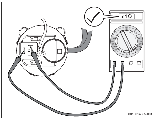
Рис. 69 Проверка проводимости дифференциального реле давления (реле в порядке)
