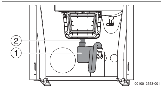
Рис. 47 Демонтаж сифона
