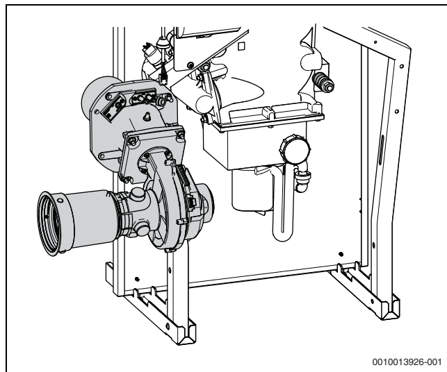
Рис. 45 Горелка в положении для обслуживания (монтаж слева)
