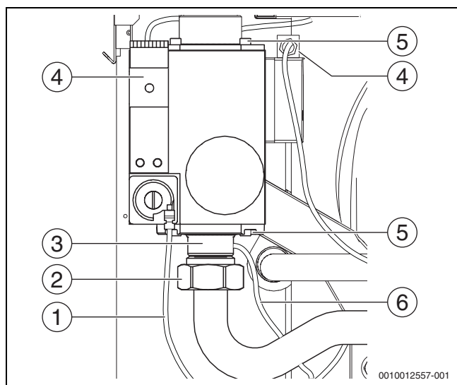
Рис. 58 Отсоединение подключений газовой арматуры (150 ... 300 кВт)
