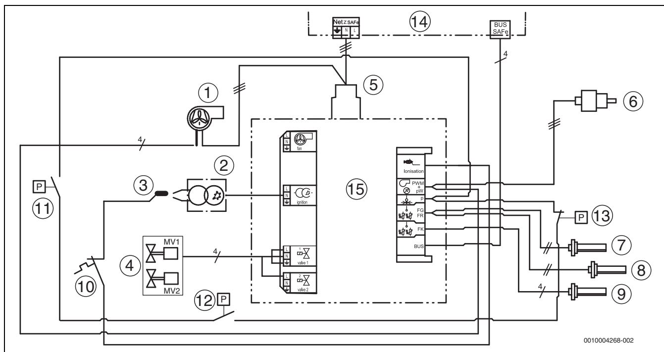
Рис. 74 Схема соединений автомата горения
