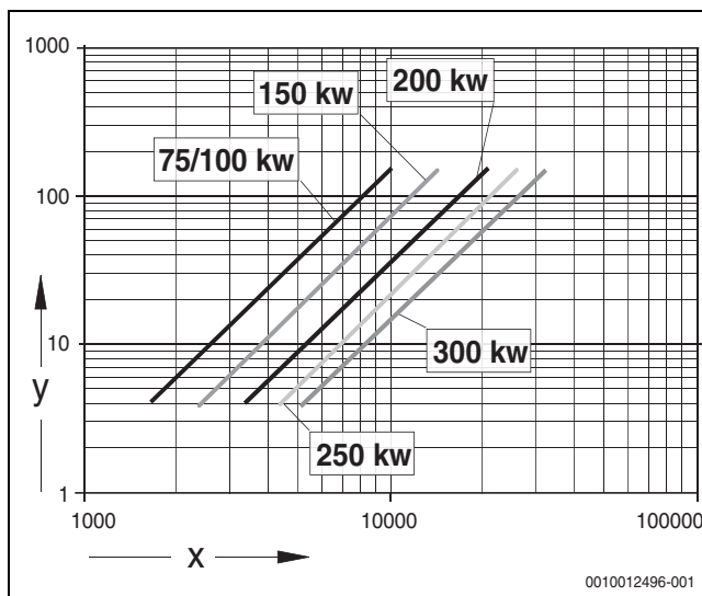
Рис. 73 Гидравлическое сопротивление греющего контура
